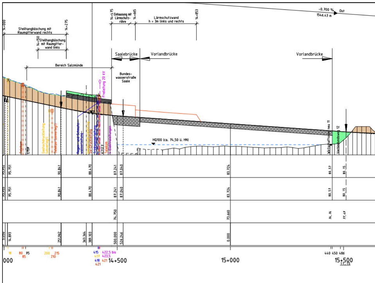
Bauwerk Saalequerung LW = 968 m (Höhenplan)
