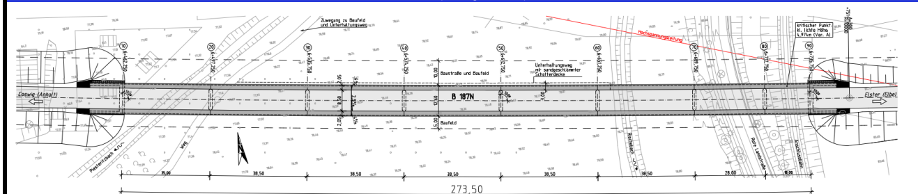
Draufsicht (Vorzugsvariante)
