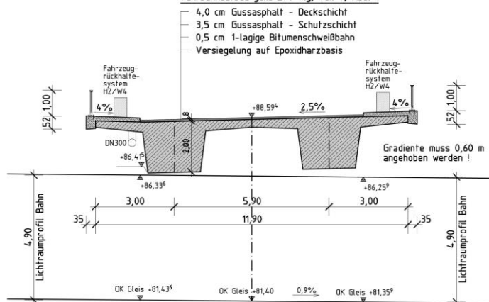
Fahrbahnaufbau gem. ZTV-Ing, Teil 7, Abs. 1
