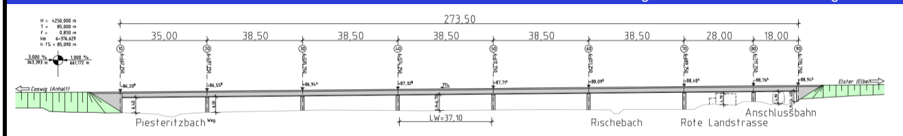
Ansicht (Vorzugsvariante)
