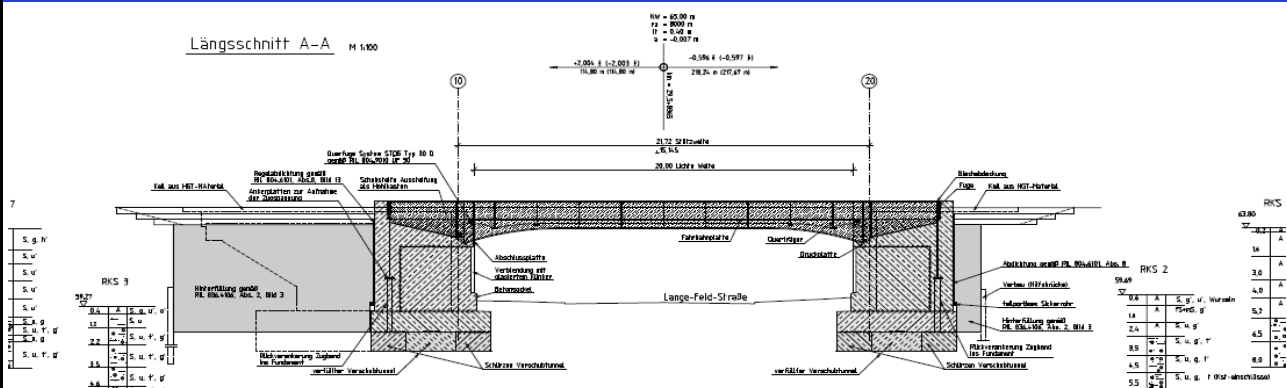
Längsschnitt
